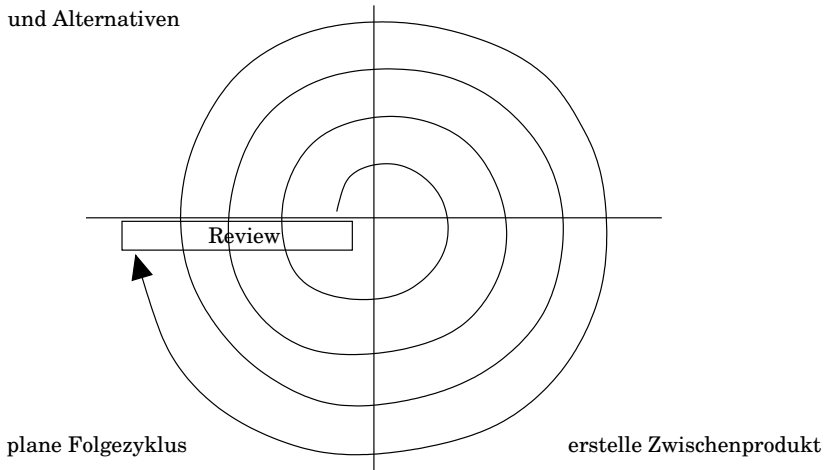
Abbildung 2: Das Spiralmodell
